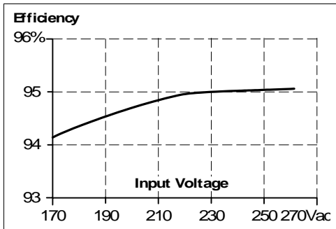
Bild 12-3 Wirkungsgrad zu Eingangsspannung bei 48V, 20A, typ.
