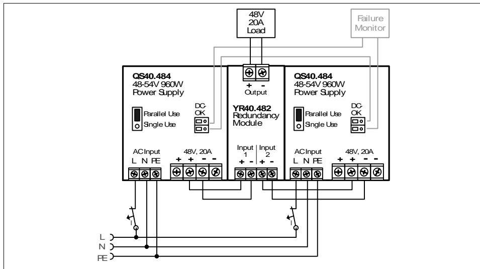
Bild 24-1 Typische 1+1 redundante Verschaltung für 20A mit einem Redundanzmodul
