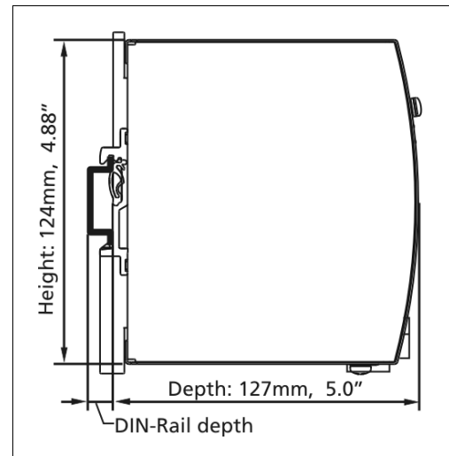
Bild 23-2 Seitenansicht
