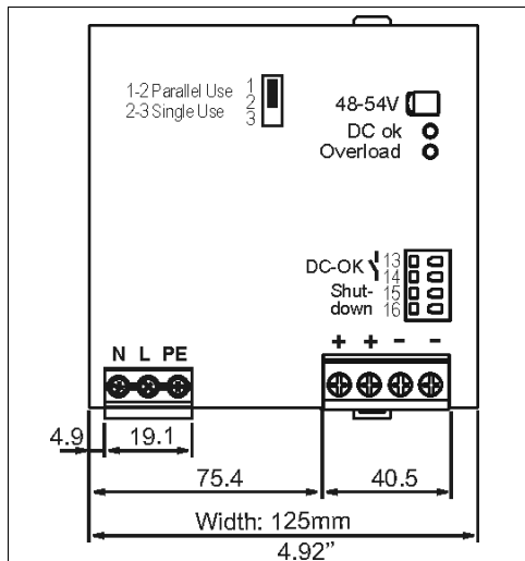
Bild 23-1 Frontansicht
