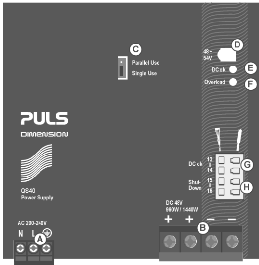
Bild 16-1 Frontseite
