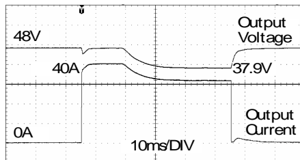
Bild 25-3 Spitzenlast mit dem zweifachen Nennstrom für 50ms, typ.
