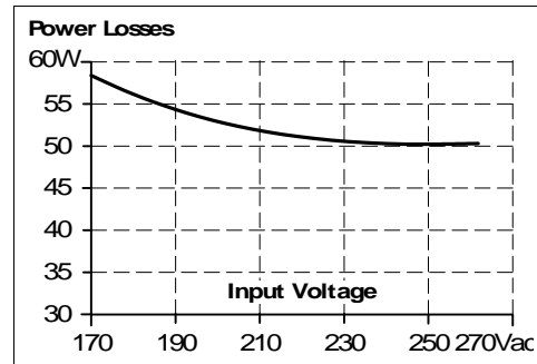
Bild 12-4 Verluste zu Eingangsspannung bei 48V, 20A, typ.
