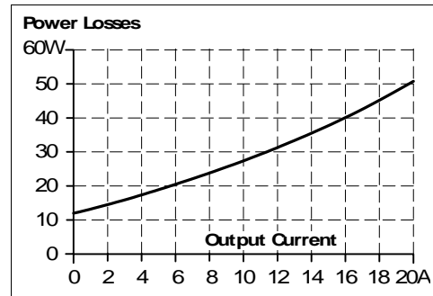
Bild 12-2 Verluste zu Ausgangsstrom bei 48V, typ.
