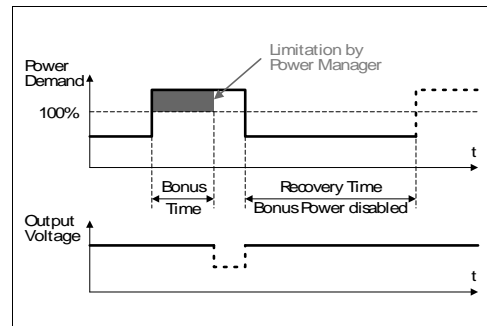
Bild 6-6 BonusPower ® -Erholzeit
