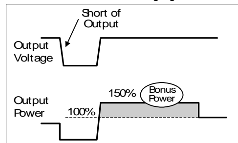
Bild 6-8 BonusPower ® nach Ausgangskurzschluss
