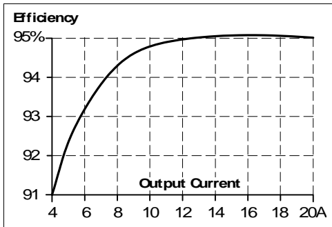
Bild 12-1 Wirkungsgrad zu Ausgangsstrom bei 48V, typ.
