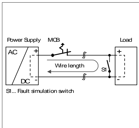
Bild 25-5 Prüfschaltung
