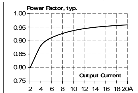
Bild 3-4 Leistungsfaktor zu Ausgangslast bei 48V
