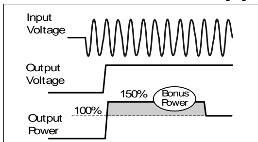
Bild 6-7 BonusPower ® nach Einschalten des Eingangs
