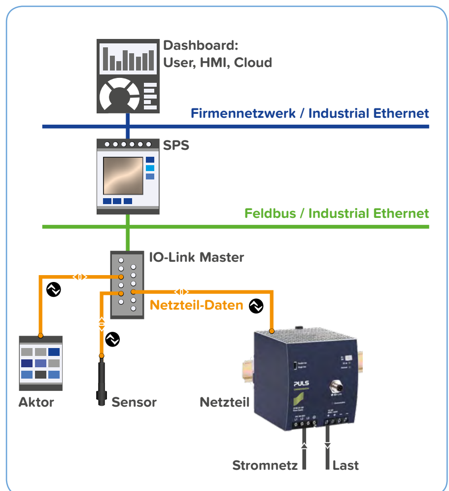
Das QT40 fügt sich über IO-Link nahtlos in die Infrastruktur ein – unabhängig vom übergeordneten Feldbus.
